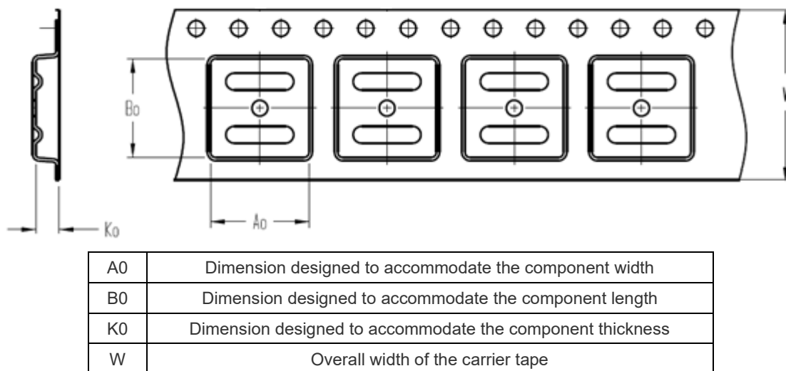
图 16 带状包装规格图
