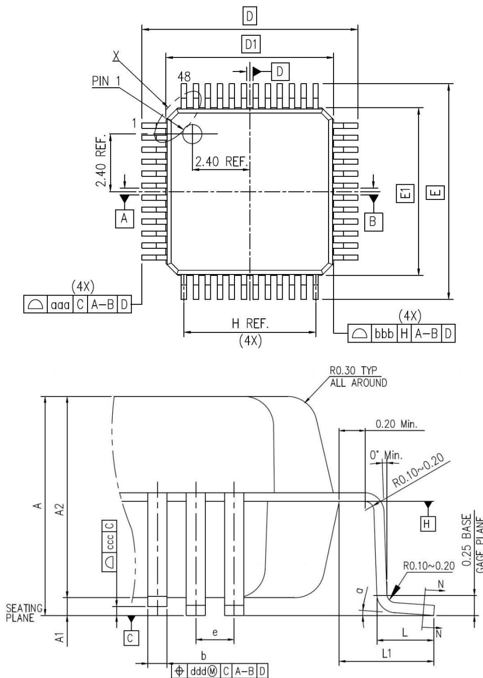
图 13 LQFP48 封装图
