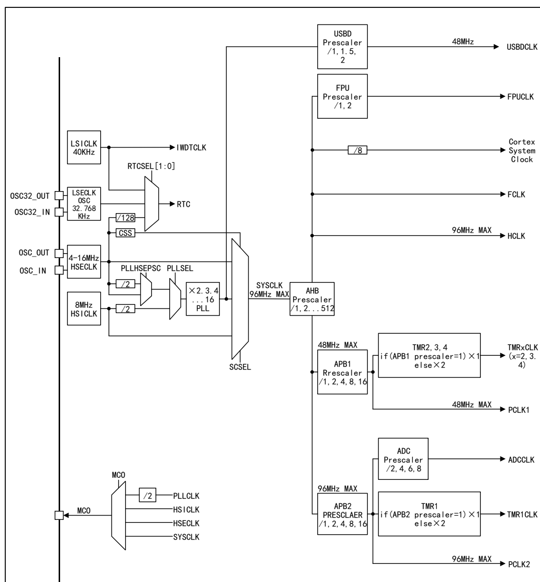
图 3 APM32A103CBT7 时钟树
